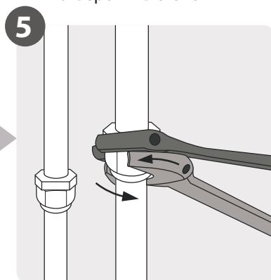
5 Соедините трубы
